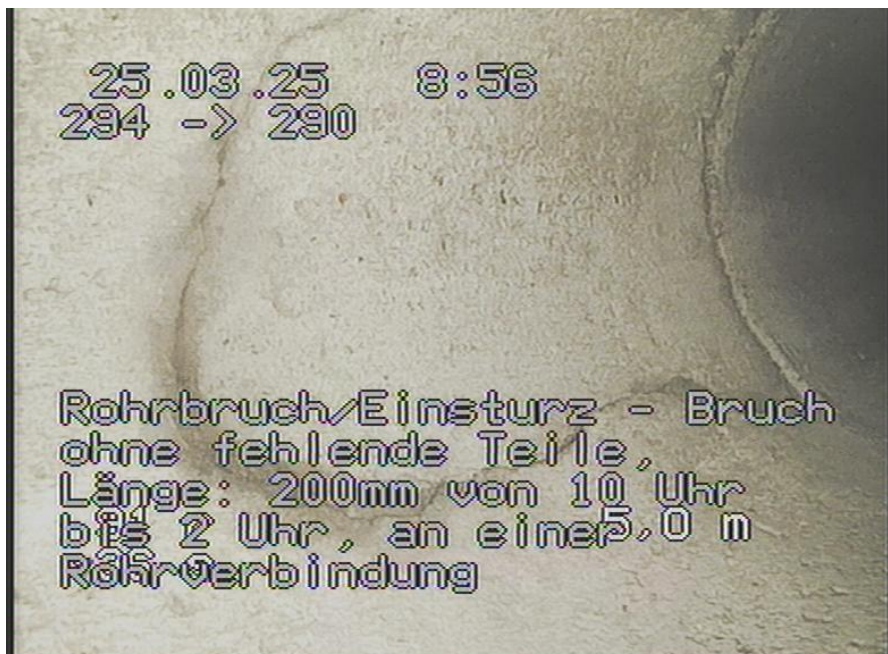
294-290_165.jpg, 00:00:38, 5.00m Rohrbruch/Einsturz - Bruch ohne fehlende Teile, Länge: 200mm von 10 Uhr bis 2 Uhr, an einer Rohrverbindung
