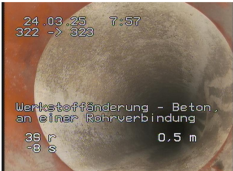
322-323_14.jpg, 00:00:20, 0.50m Werkstoffänderung - Beton, an einer Rohrverbindung
