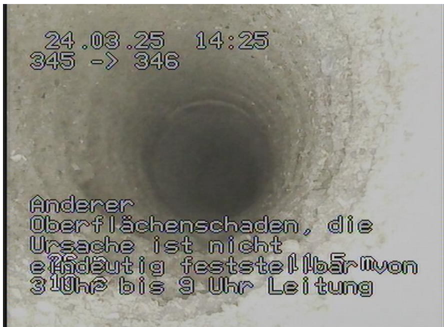
345-346_118.jpg, 00:01:32, 11.50m Anderer Oberflächenschaden, die Ursache ist nicht eindeutig feststellbar von 3 Uhr bis 9 Uhr / Leitung stark ausgespült
