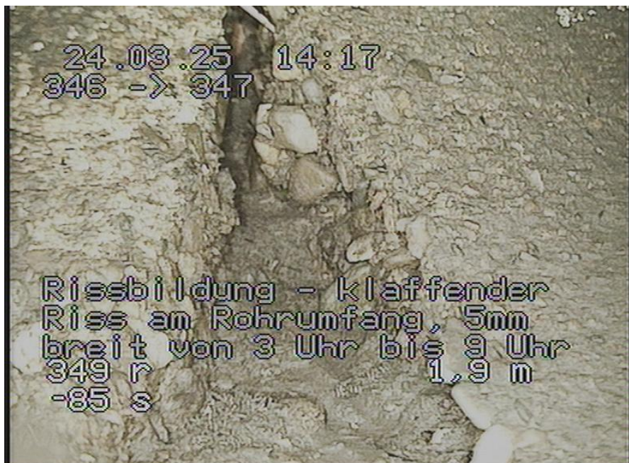
346-347_114.jpg, 00:00:32, 1.90m Rissbildung - klaffender Riss am Rohrumfang, 5mm breit von 3 Uhr bis 9 Uhr
