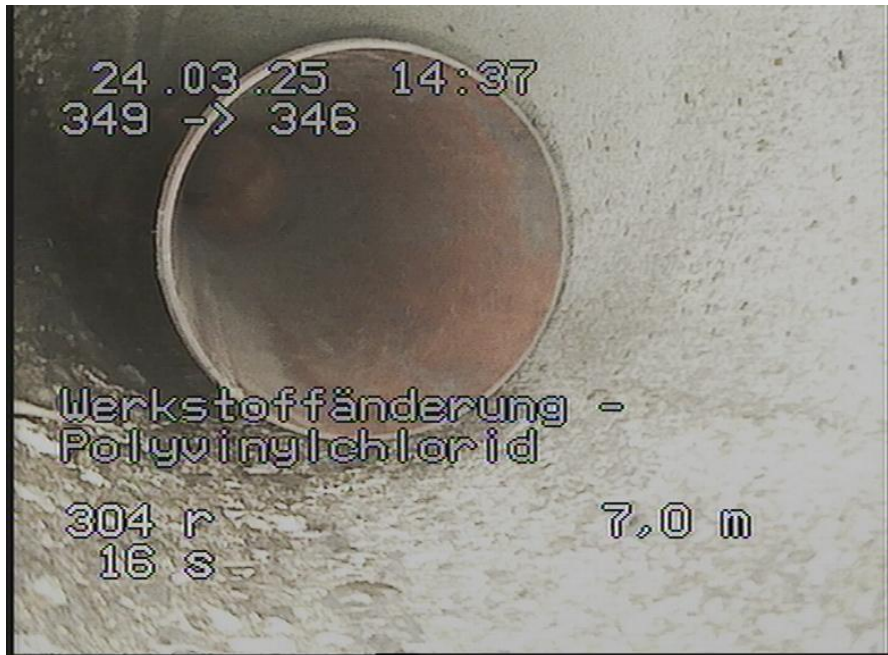
349-346_126.jpg, 00:01:20, 7.00m Werkstoffänderung - Polyvinylchlorid
