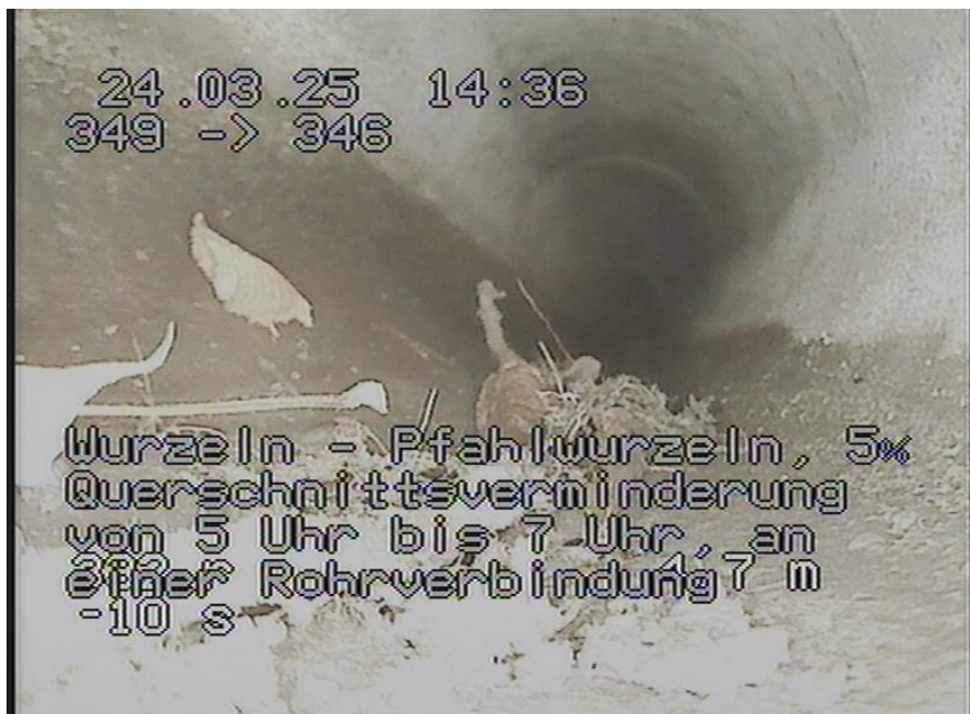
349-346_125.jpg, 00:00:52, 4.70m Wurzeln - Pfahlwurzeln, 5% Querschnittsverminderung von 5 Uhr bis 7 Uhr, an einer Rohrverbindung
