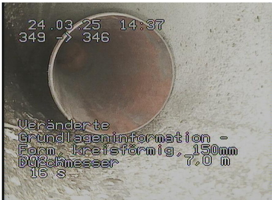
349-346_127.jpg, 00:01:24, 7.00m Veränderte Grundlageninformation - Form, kreisförmig, 150mm Durchmesser
