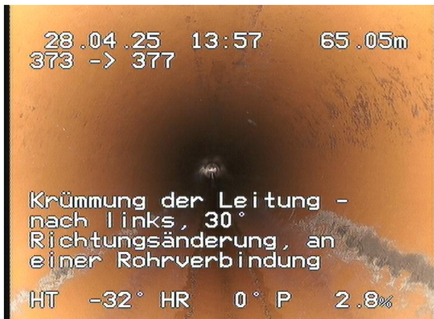
373-377_399.jpg, 00:04:28, 65.05m Krümmung der Leitung - nach links, 30° Richtungsänderung, an einer Rohrverbindung
