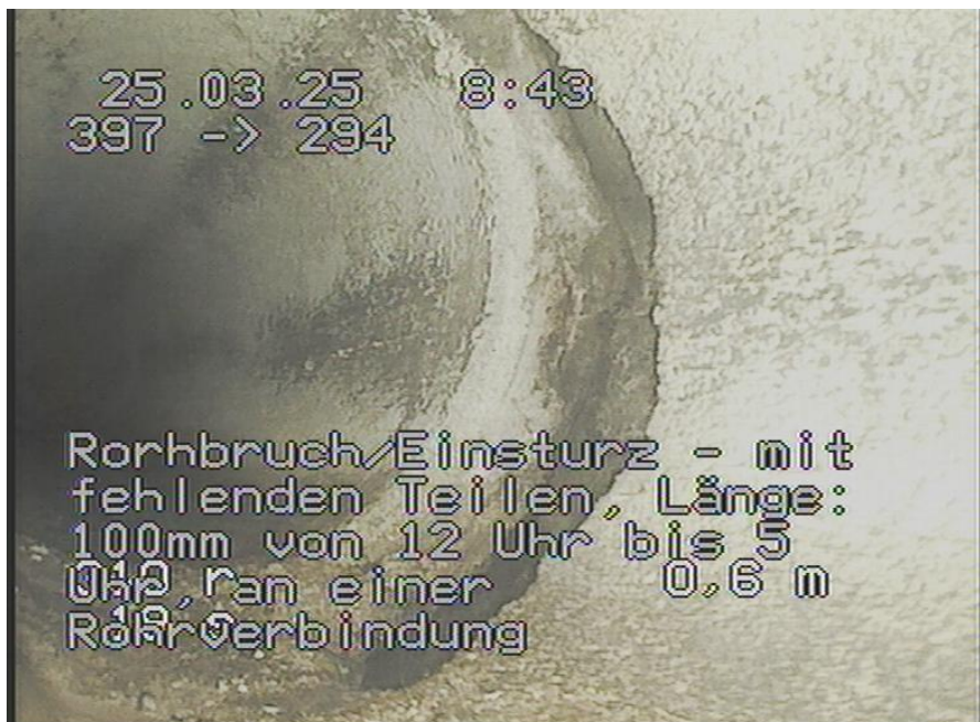
397-294_159.jpg, 00:00:24, 0.60m Rohrbruch/Einsturz - mit fehlenden Teilen, Länge: 100mm von 12 Uhr bis 5 Uhr, an einer Rohrverbindung
