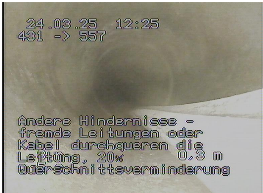
431-557_74.jpg, 00:02:52, 0.01m Andere Hindernisse - fremde Leitungen oder Kabel durchqueren die Leitung, 20% Querschnittsverminderung von 3 Uhr bis 6 Uhr, Anfang
