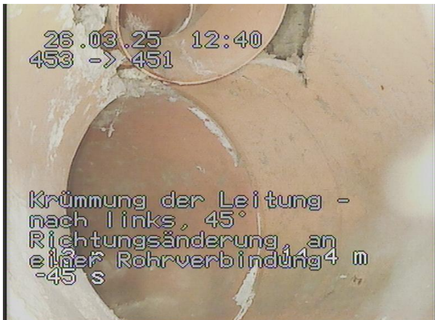
453-451_284.jpg, 00:00:50, 14.40m Krümmung der Leitung - nach links, 45° Richtungsänderung, an einer Rohrverbindung
