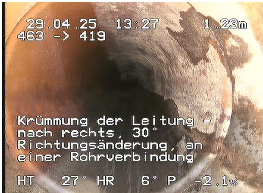
463-419_457.jpg, 00:00:19, 1.23m Krümmung der Leitung - nach rechts, 30° Richtungsänderung, an einer Rohrverbindung
