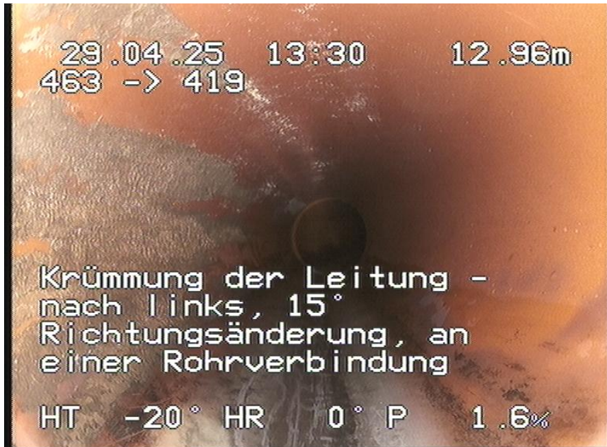
463-419_460.jpg, 00:02:19, 12.96m Krümmung der Leitung - nach links, 15° Richtungsänderung, an einer Rohrverbindung
