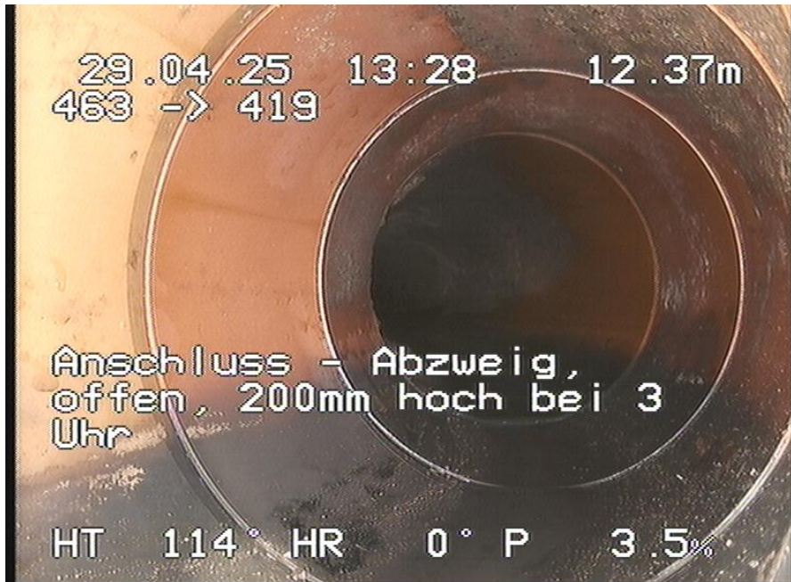
463-419_458.jpg, 00:01:16, 12.37m Anschluss - Abzweig, offen, 200mm hoch bei 3 Uhr
