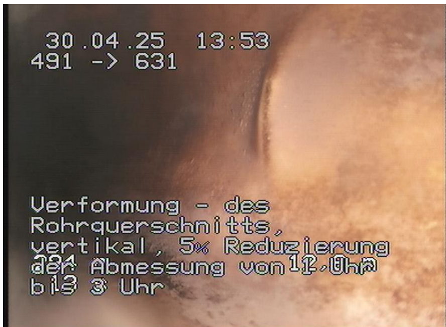
491-631_514.jpg, 00:03:50, 12.60m Verformung - des Rohrquerschnitts, vertikal, 5% Reduzierung der Abmessung von 1 Uhr bis 3 Uhr
