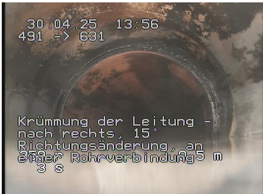
491-631_516.jpg, 00:05:18, 0.50m Krümmung der Leitung - nach rechts, 15° Richtungsänderung, an einer Rohrverbindung
