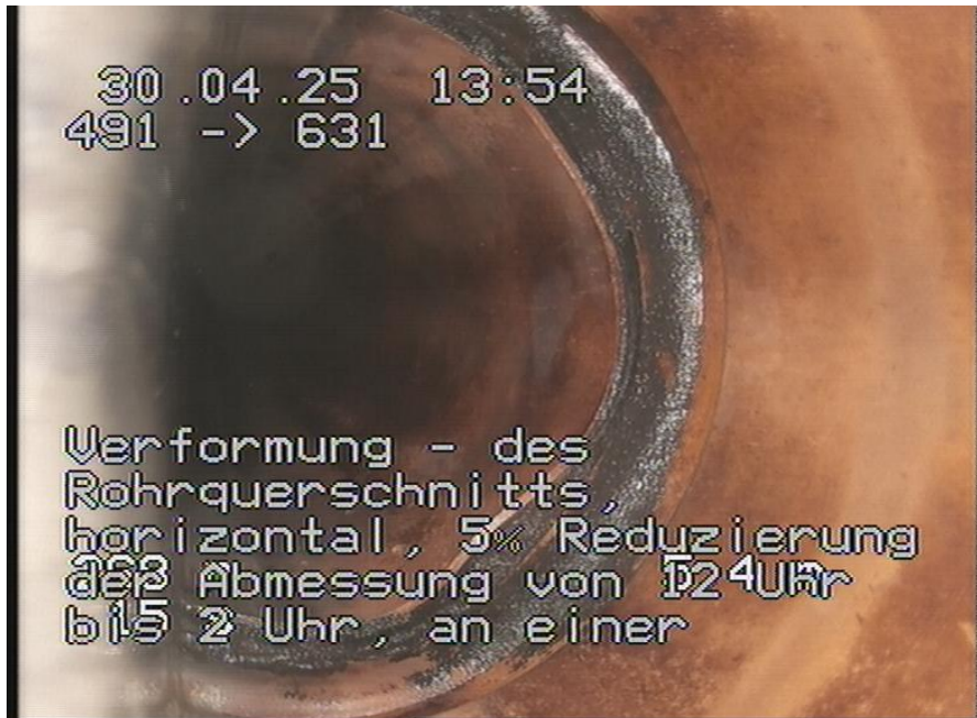
491-631_515.jpg, 00:04:33, 5.40m Verformung - des Rohrquerschnitts, horizontal, 5% Reduzierung der Abmessung von 12 Uhr bis 2 Uhr, an einer Rohrverbindung
