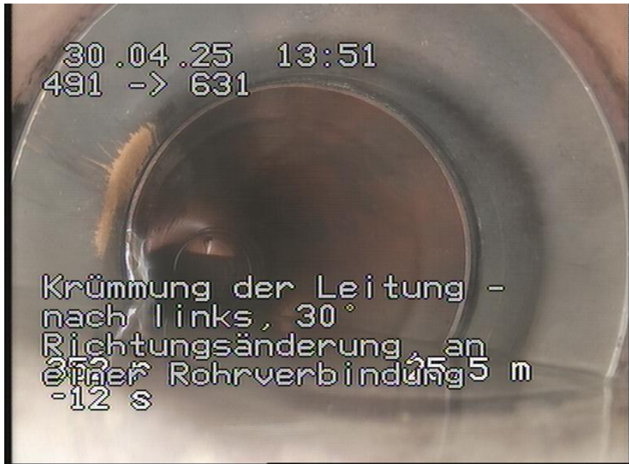
491-631_512.jpg, 00:02:27, 25.50m Krümmung der Leitung - nach links, 30° Richtungsänderung, an einer Rohrverbindung
