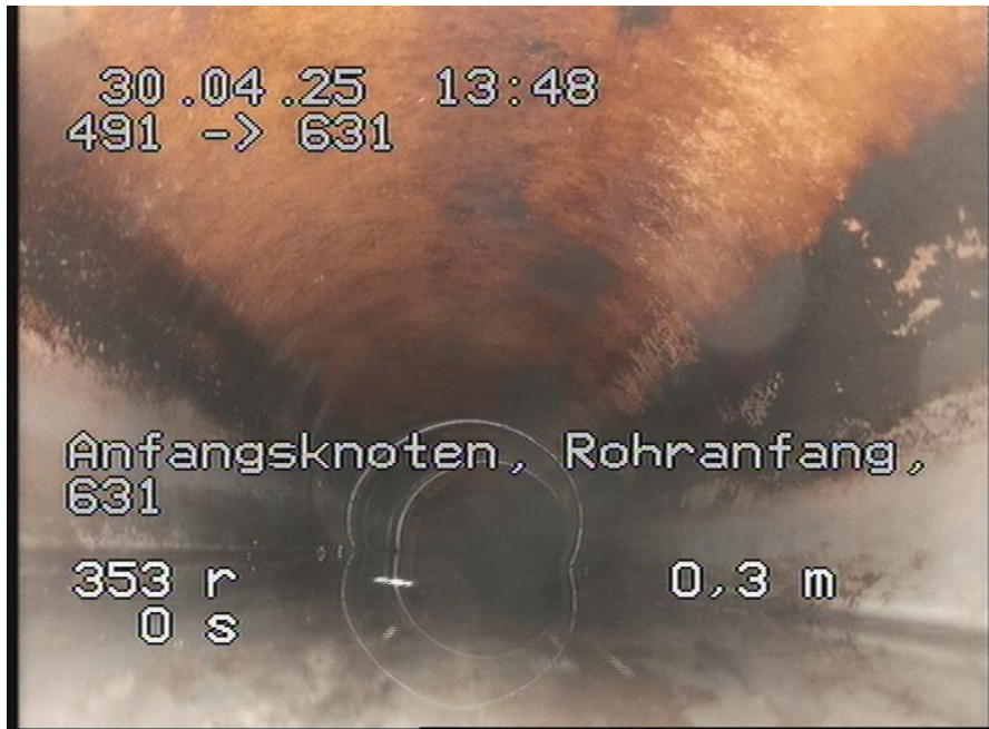
491-631_511.jpg, 00:00:00, 0.00m Anfangsknoten, Rohranfang, 631
