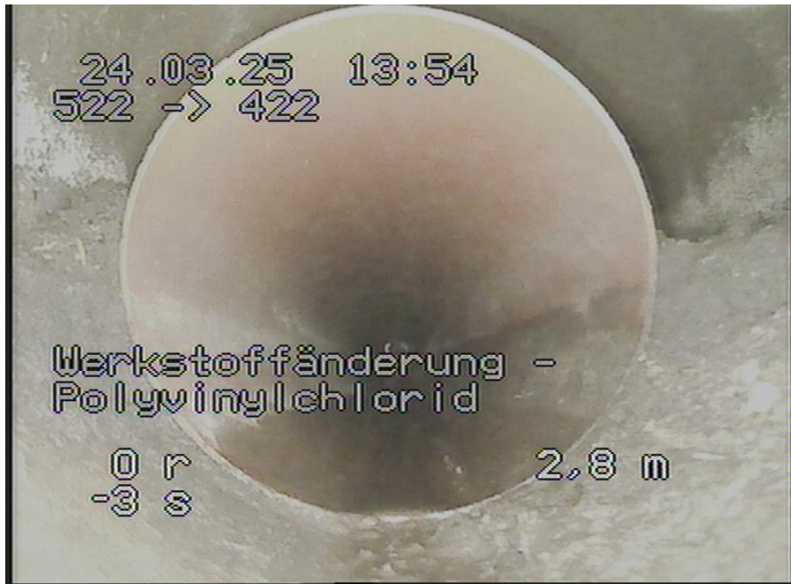
522-422_109.jpg, 00:00:39, 2.80m Werkstoffänderung - Polyvinylchlorid
