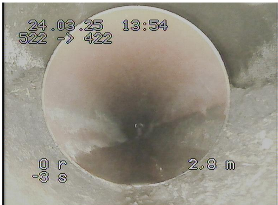
522-422_108.jpg, 00:00:32, 2.80m Veränderte Grundlageninformation - Form, kreisförmig, 150mm Durchmesser
