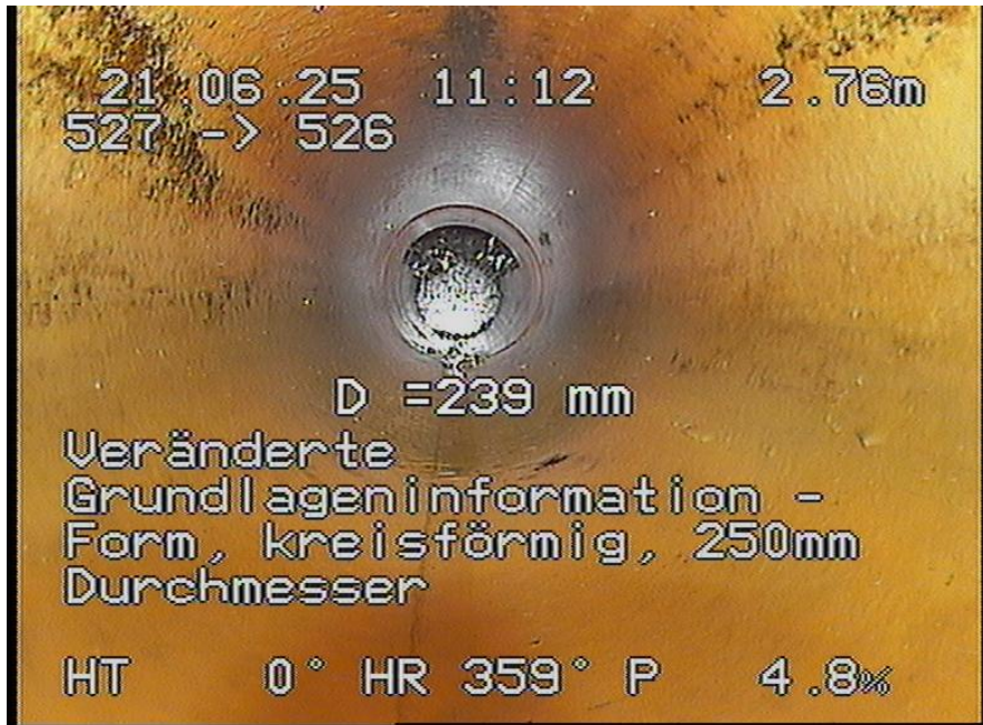
527-526_731.jpg, 00:01:39, 2.37m Veränderte Grundlageninformation - Form, kreisförmig, 250mm Durchmesser
