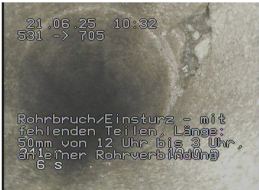
531-705_723.jpg, 00:00:57, 10.00m Rohrbruch/Einsturz - mit fehlenden Teilen, Länge: 50mm von 12 Uhr bis 3 Uhr, an einer Rohrverbindung
