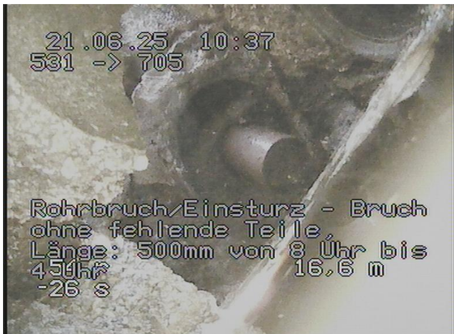
531-705_727.jpg, 00:02:32, 16.60m Rohrbruch/Einsturz - Bruch ohne fehlende Teile, Länge: 500mm von 8 Uhr bis 4 Uhr
