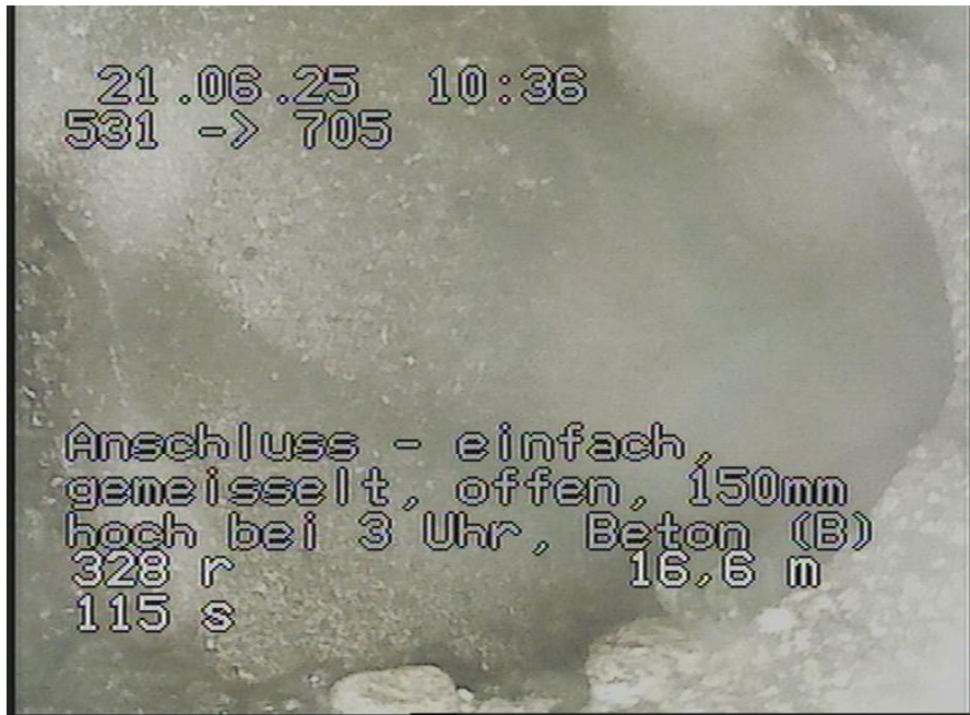
531-705_726.jpg, 00:02:28, 16.60m Anschluss - einfach, gemeisselt, offen, 150mm hoch bei 3 Uhr, Beton (B)
