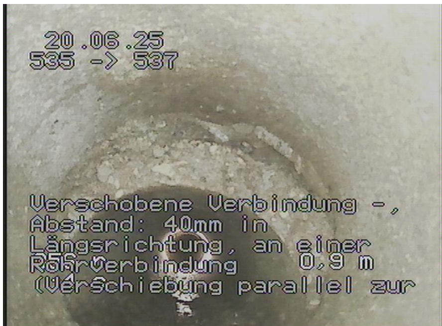
535-537_674.jpg, 00:00:20, 0.90m Verschobene Verbindung -, Abstand: 40mm in Längsrichtung, an einer Rohrverbindung (Verschiebung parallel zur Rohrachse) von 9 Uhr bis 3 Uhr
