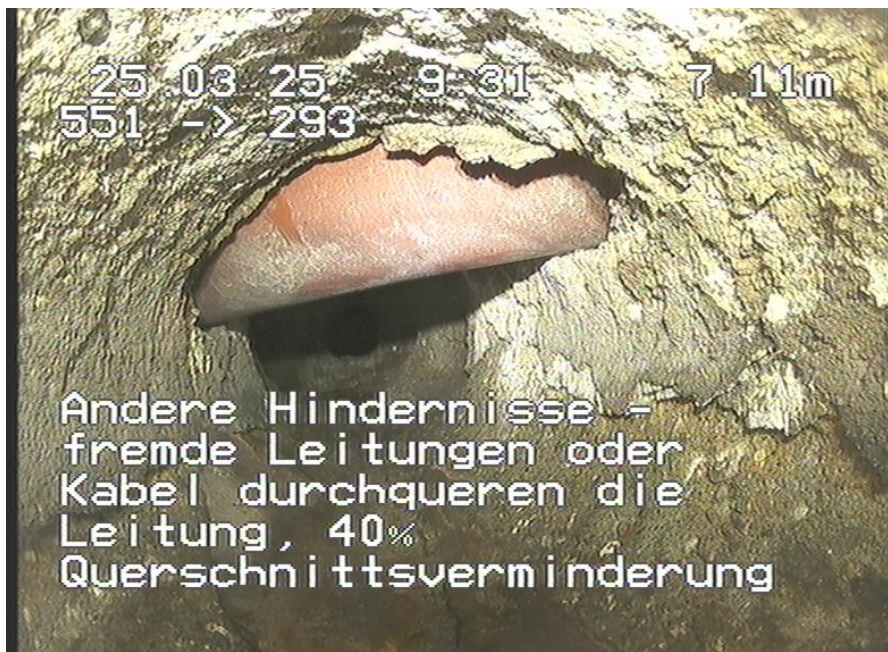
551-293_179.jpg, 00:01:55, 7.11m Andere Hindernisse - fremde Leitungen oder Kabel durchqueren die Leitung, 40% Querschnittsverminderung von 10 Uhr bis 2 Uhr
