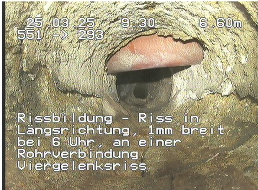
551-293_178.jpg, 00:01:34, 6.59m Rissbildung - Riss in Längsrichtung, 1mm breit bei 6 Uhr, an einer Rohrverbindung / Viergelenksriss
