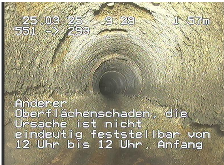
551-293_177.jpg, 00:00:34, 1.57m Anderer Oberflächenschaden, die Ursache ist nicht eindeutig feststellbar von 12 Uhr bis 12 Uhr, Anfang
