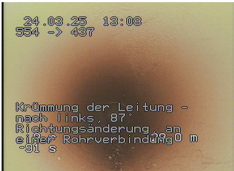
554-437_99.jpg, 00:02:26, 28.00m Krümmung der Leitung - nach links, 87° Richtungsänderung, an einer Rohrverbindung
