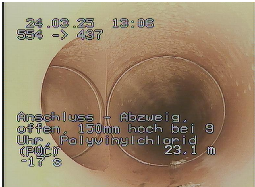
554-437_97.jpg, 00:01:20, 23.10m Anschluss - Abzweig, offen, 100mm hoch bei 9 Uhr, Polyvinylchlorid (PVC)
