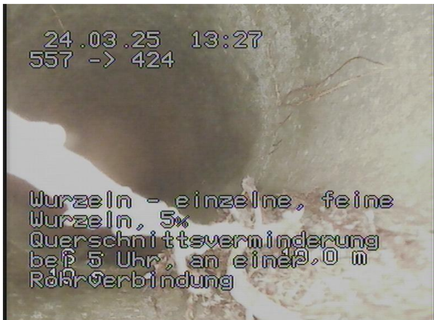
557-424_102.jpg, 00:00:42, 10.00m Wurzeln - einzelne, feine Wurzeln, 5% Querschnittsverminderung bei 5 Uhr, an einer Rohrverbindung
