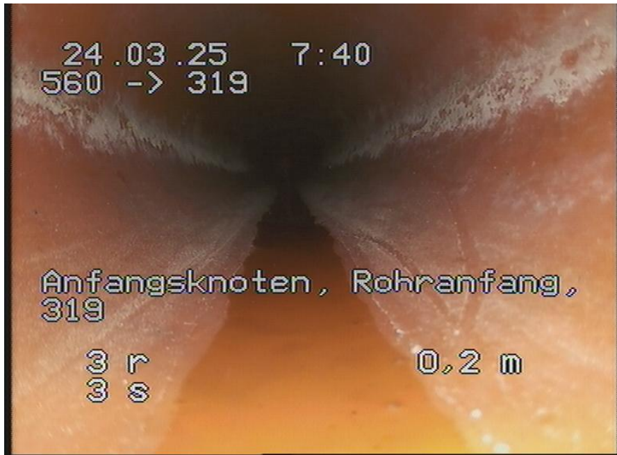
560-319_1.jpg, 00:00:00, 0.00m Anfangsknoten, Rohranfang, 319
