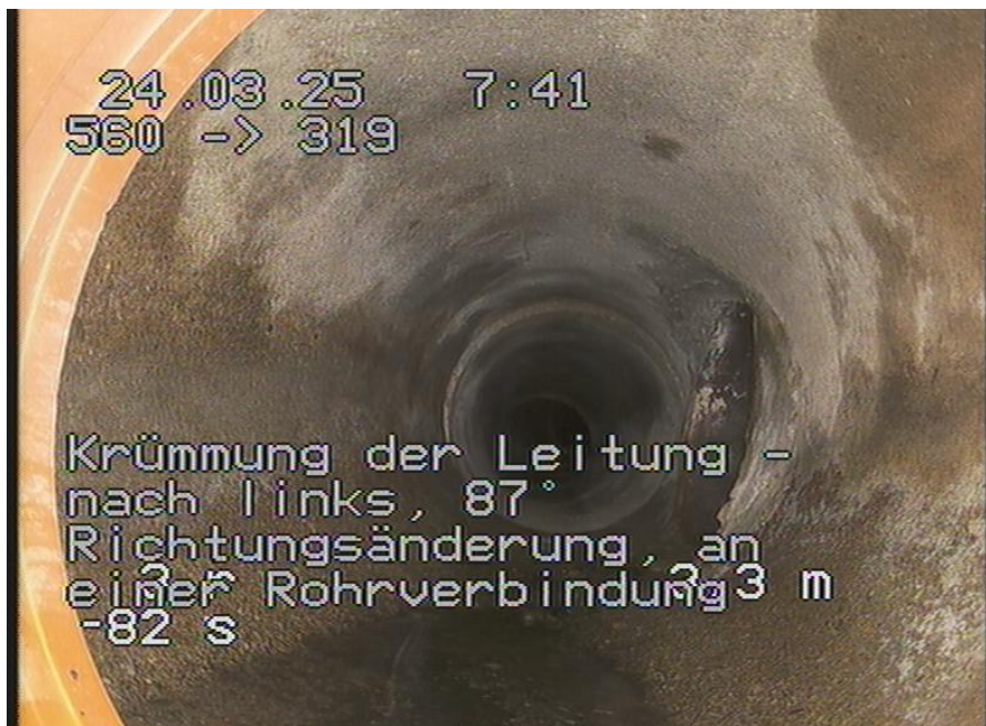
560-319_2.jpg, 00:00:33, 3.30m Krümmung der Leitung - nach links, 87° Richtungsänderung, an einer Rohrverbindung
