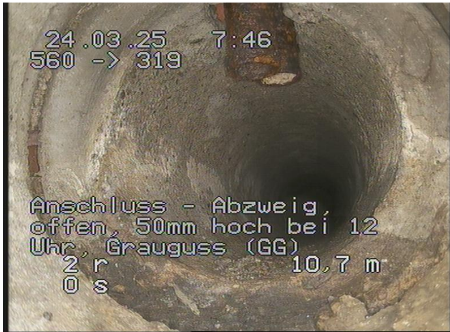
560-319_7.jpg, 00:02:41, 10.70m Anschluss - Abzweig, offen, 50mm hoch bei 12 Uhr, Grauguss (GG)
