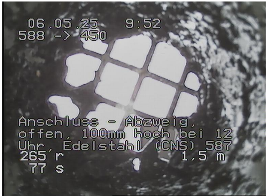
588-450_537.jpg, 00:00:41, 1.50m Anschluss - Abzweig, offen, 100mm hoch bei 12 Uhr, Edelstahl (CNS) / 587
