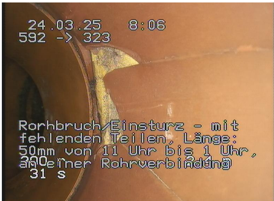
592-323_19.jpg, 00:00:40, 2.40m Rohrbruch/Einsturz - mit fehlenden Teilen, Länge: 50mm von 11 Uhr bis 1 Uhr, an einer Rohrverbindung
