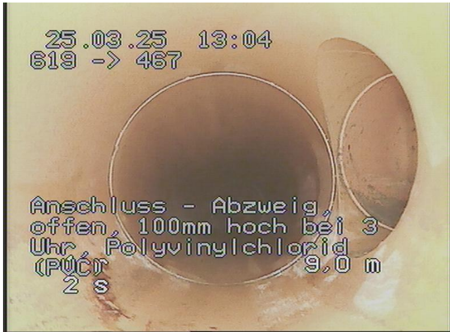
619-467_244.jpg, 00:01:02, 9.00m Anschluss - Abzweig, offen, 100mm hoch bei 3 Uhr, Polyvinylchlorid (PVC)
