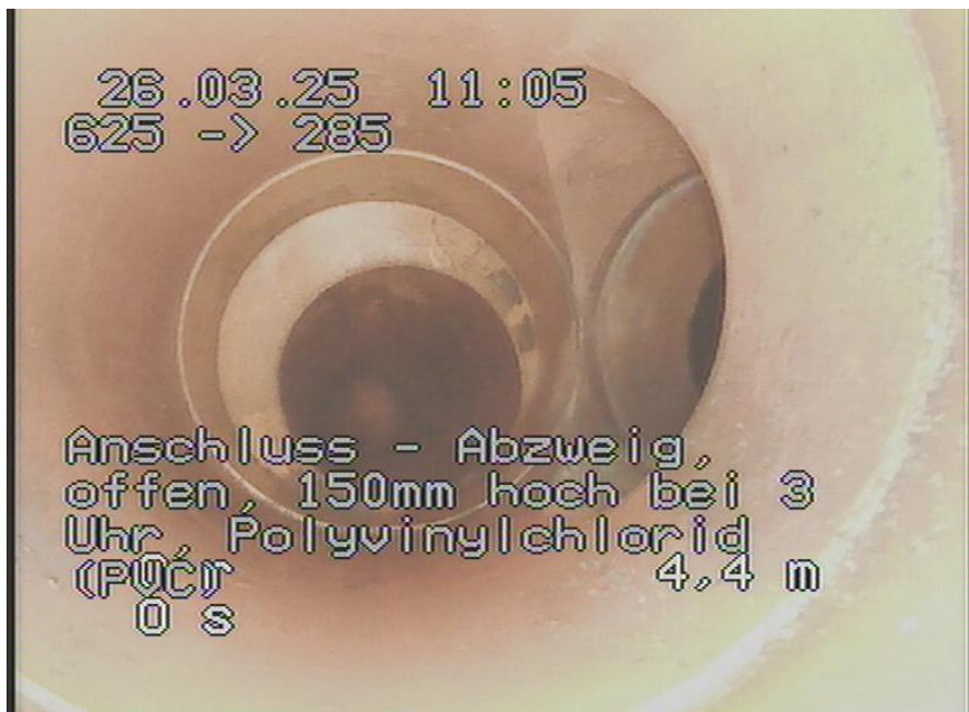
625-285_266.jpg, 00:00:32, 4.40m Anschluss - Abzweig, offen, 150mm hoch bei 3 Uhr, Polyvinylchlorid (PVC)
