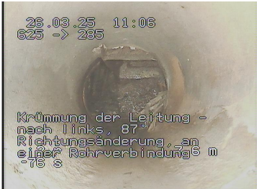
625-285_269.jpg, 00:01:22, 7.60m Krümmung der Leitung - nach links, 87° Richtungsänderung, an einer Rohrverbindung
