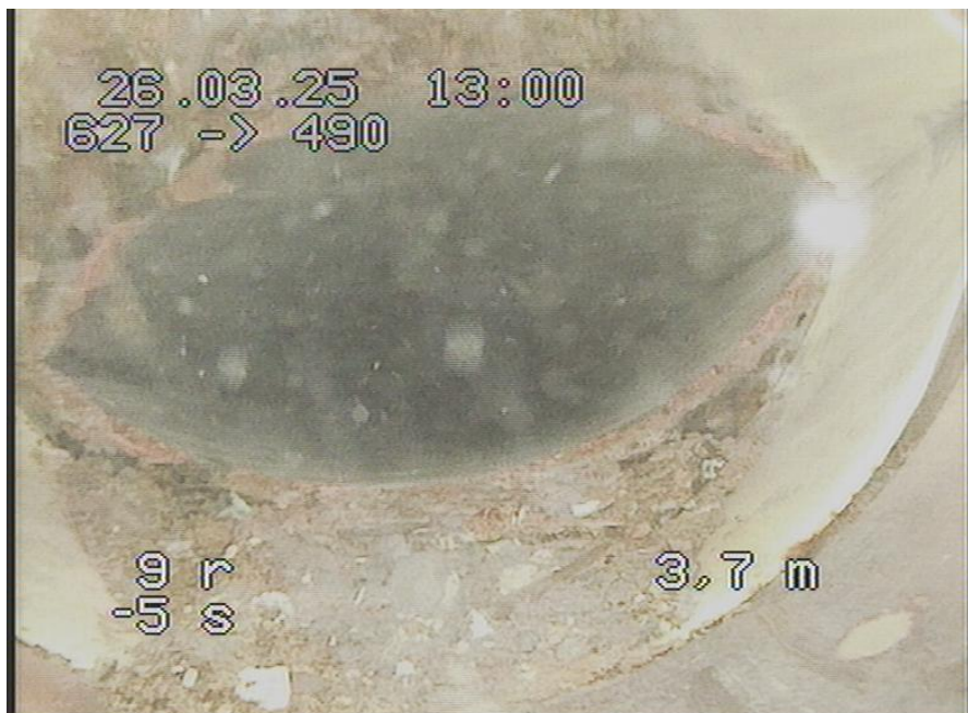
627-490_287.jpg, 00:00:29, 3.70m Verschobene Verbindung -, Versatz: 20mm rechtwinklig zur Rohrachse, an einer Rohrverbindung von 3 Uhr bis 9 Uhr
