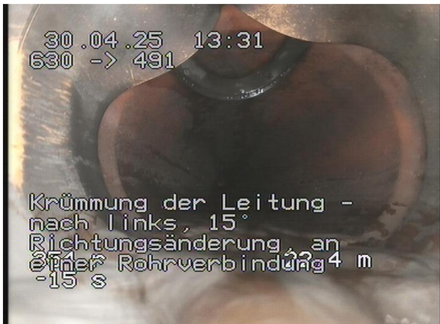
630-491_507.jpg, 00:01:55, 22.40m Krümmung der Leitung - nach links, 15° Richtungsänderung, an einer Rohrverbindung
