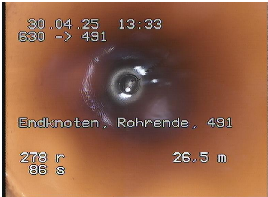
630-491_510.jpg, 00:02:47, 26.60m Endknoten, Rohrende, 491
