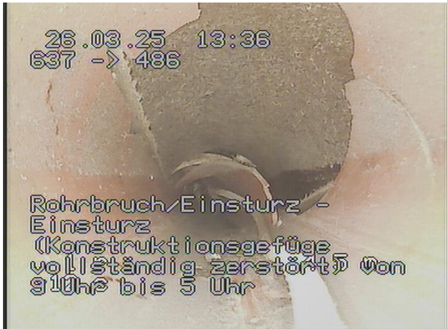
637-486_297.jpg, 00:00:53, 5.00m Rohrbruch/Einsturz - Einsturz (Konstruktionsgefüge vollständig zerstört) von 9 Uhr bis 5 Uhr
