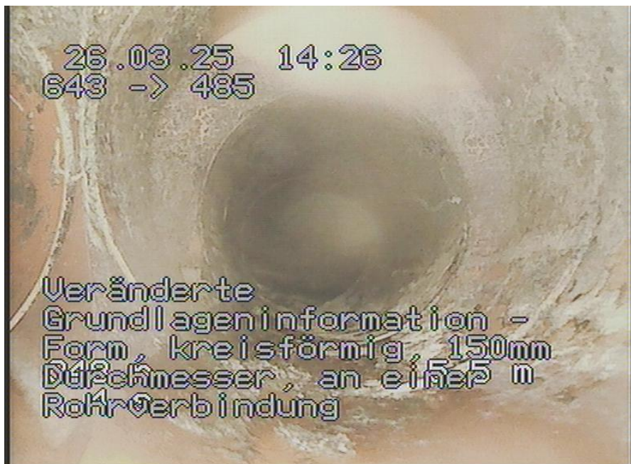
643-485_321.jpg, 00:02:00, 5.50m Veränderte Grundlageninformation - Form, kreisförmig, 150mm Durchmesser, an einer Rohrverbindung
