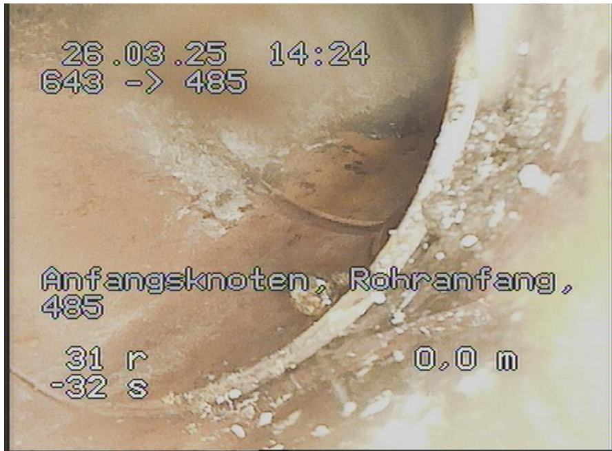
643-485_318.jpg, 00:00:00, 0.00m Anfangsknoten, Rohranfang, 485
