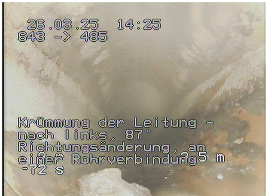
643-485_319.jpg, 00:01:29, 3.50m Krümmung der Leitung - nach links, 87° Richtungsänderung, an einer Rohrverbindung
