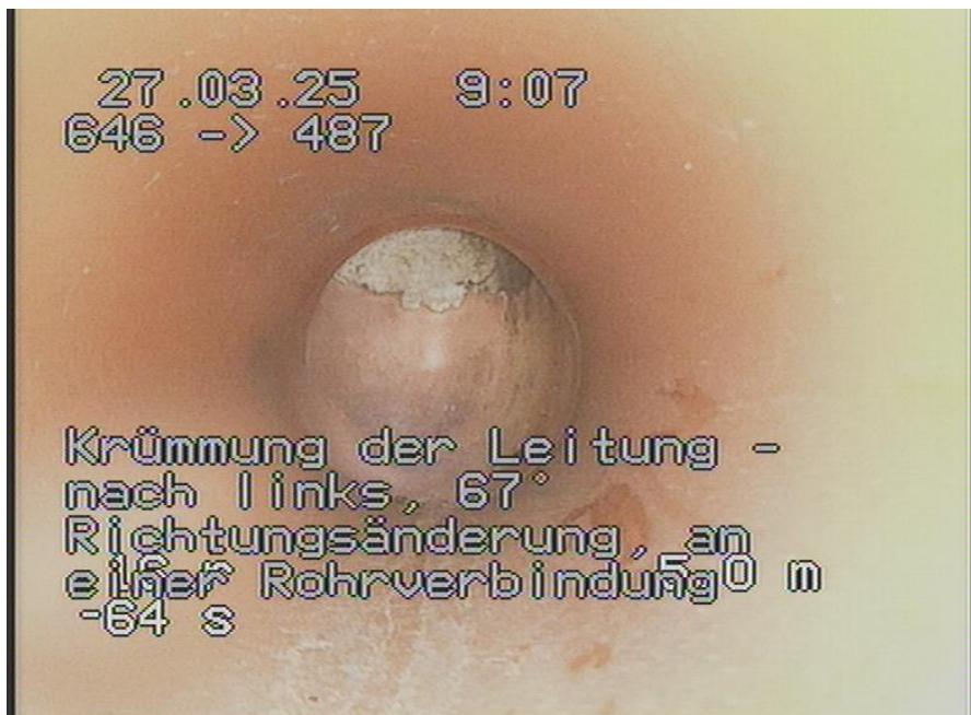
646-487_350.jpg, 00:00:58, 5.00m Krümmung der Leitung - nach links, 67° Richtungsänderung, an einer Rohrverbindung
