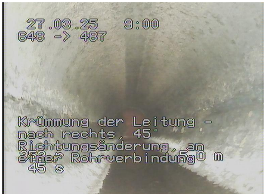
648-487_342.jpg, 00:01:47, 5.00m Krümmung der Leitung - nach rechts, 45° Richtungsänderung, an einer Rohrverbindung
