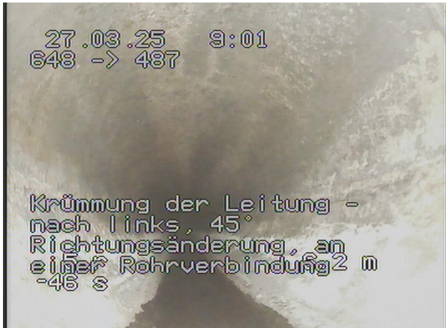
648-487_343.jpg, 00:02:00, 6.20m Krümmung der Leitung - nach links, 45° Richtungsänderung, an einer Rohrverbindung
