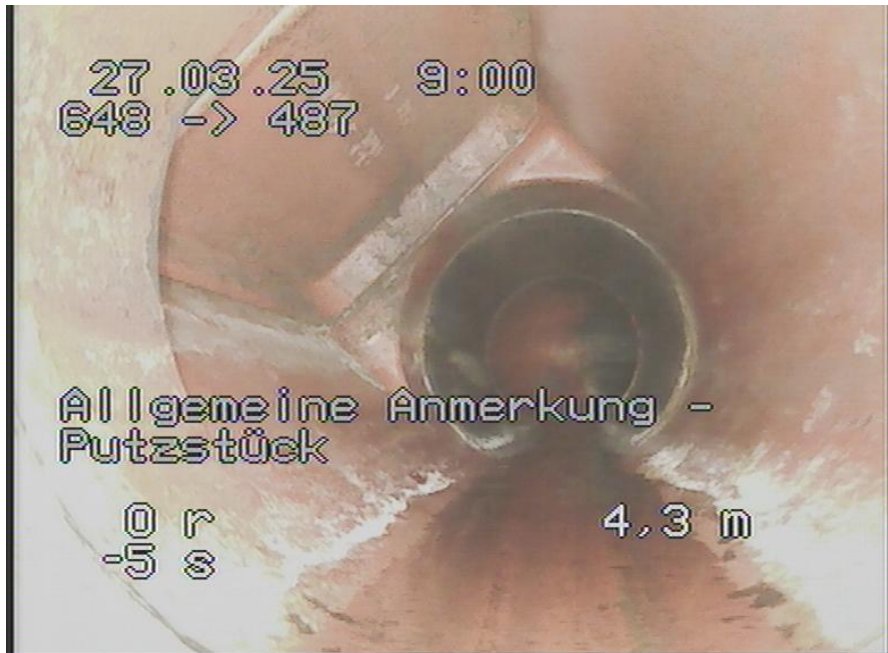
648-487_341.jpg, 00:01:32, 4.30m Allgemeine Anmerkung - / Putzstück
