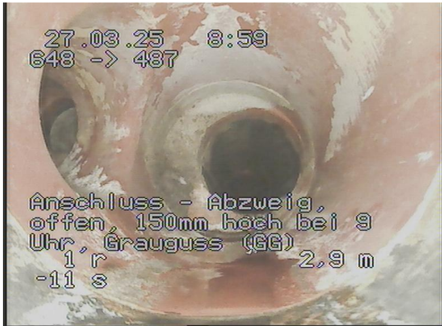
648-487_339.jpg, 00:01:05, 2.90m Anschluss - Abzweig, offen, 150mm hoch bei 9 Uhr, Grauguss (GG)
