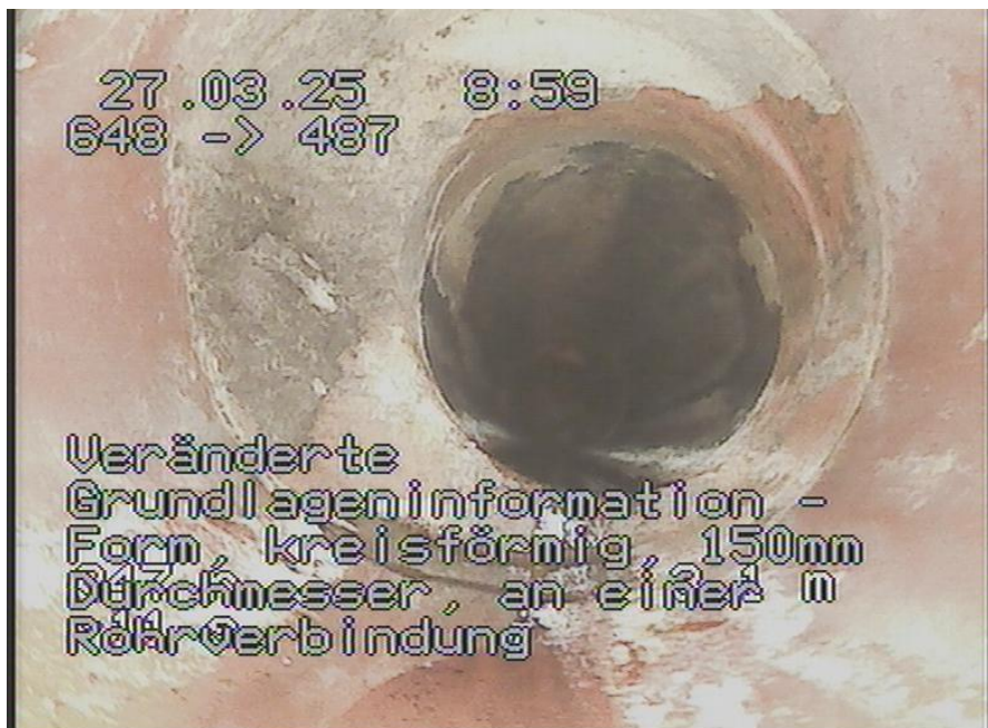
648-487_340.jpg, 00:01:17, 3.10m Veränderte Grundlageninformation - Form, kreisförmig, 150mm Durchmesser, an einer Rohrverbindung
