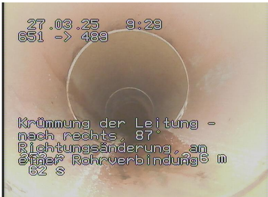
651-489_355.jpg, 00:00:36, 2.60m Krümmung der Leitung - nach rechts, 87° Richtungsänderung, an einer Rohrverbindung
