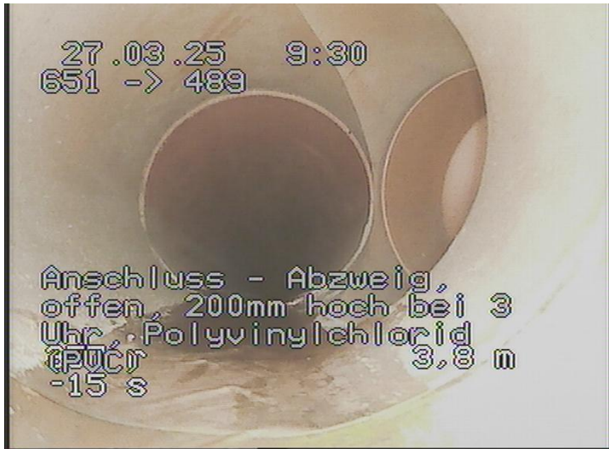
651-489_356.jpg, 00:00:58, 3.80m Anschluss - Abzweig, offen, 200mm hoch bei 3 Uhr, Polyvinylchlorid (PVC)
