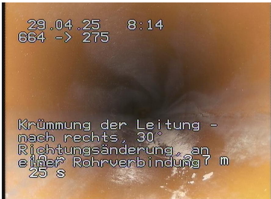
664-275_406.jpg, 00:00:26, 3.70m Krümmung der Leitung - nach rechts, 30° Richtungsänderung, an einer Rohrverbindung
