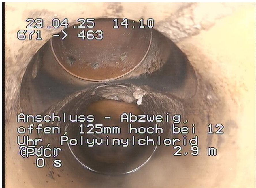
671-463_470.jpg, 00:00:33, 2.90m Anschluss - Abzweig, offen, 125mm hoch bei 12 Uhr, Polyvinylchlorid (PVC)
