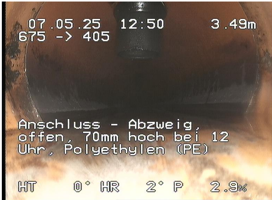
675-405_606.jpg, 00:00:49, 3.49m Anschluss - Abzweig, offen, 70mm hoch bei 12 Uhr, Polyethylen (PE)
