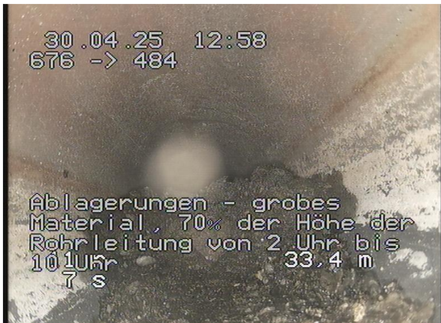
676-484_493.jpg, 00:03:55, 33.40m Ablagerungen - grobes Material, 70% der Höhe der Rohrleitung von 2 Uhr bis 10 Uhr
