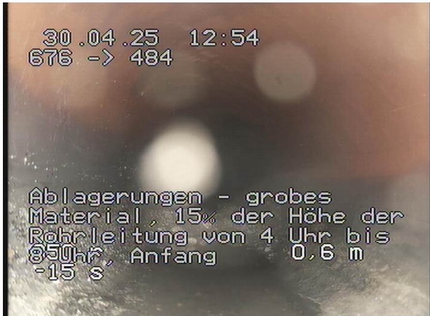
676-484_490.jpg, 00:01:02, 0.60m Ablagerungen - grobes Material, 15% der Höhe der Rohrleitung von 4 Uhr bis 8 Uhr, Anfang
