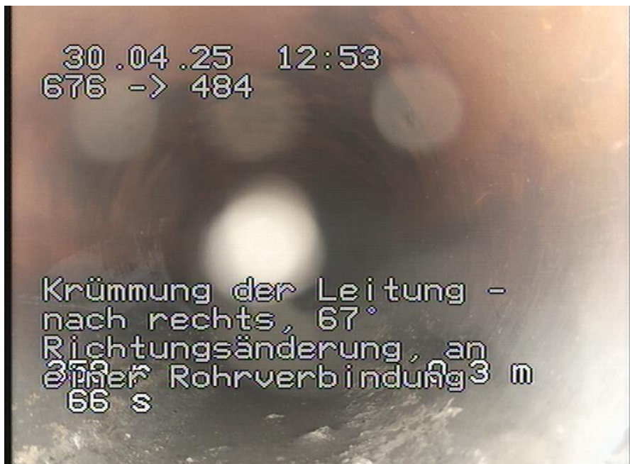
676-484_489.jpg, 00:00:43, 0.30m Krümmung der Leitung - nach rechts, 67° Richtungsänderung, an einer Rohrverbindung
