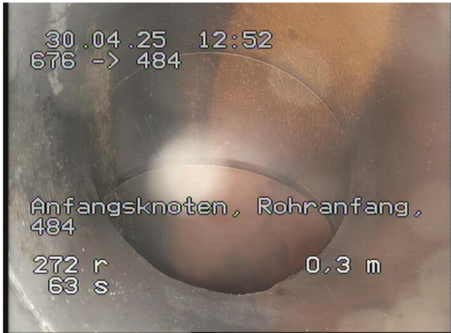
676-484_488.jpg, 00:00:00, 0.00m Anfangsknoten, Rohranfang, 484
