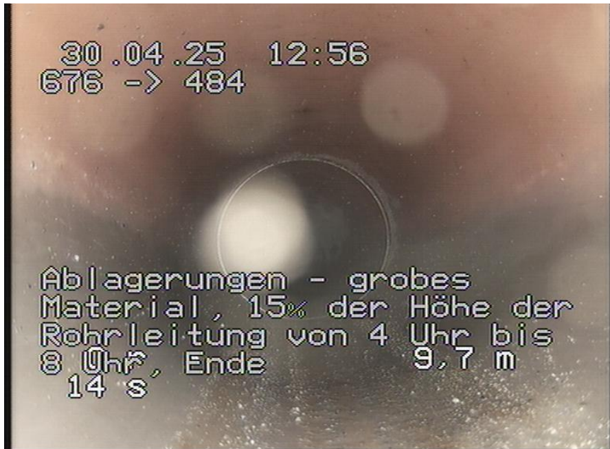
676-484_492.jpg, 00:02:33, 9.70m Ablagerungen - grobes Material, 15% der Höhe der Rohrleitung von 4 Uhr bis 8 Uhr, Ende
