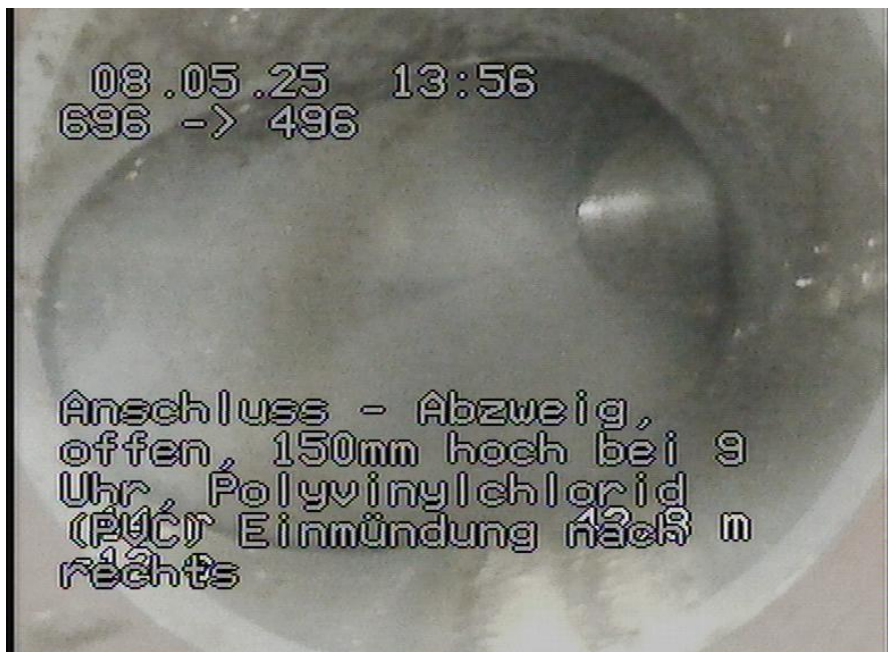
696-496_668.jpg, 00:05:52, 42.80m Anschluss - Abzweig, offen, 150mm hoch bei 9 Uhr, Polyvinylchlorid (PVC) / Einmündung nach rechts
