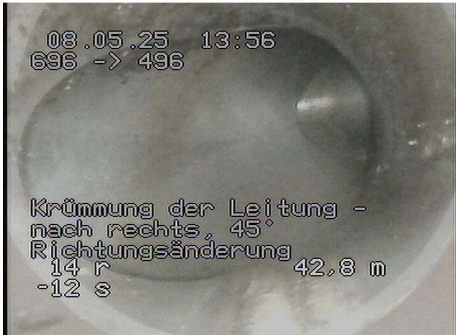
696-496_667.jpg, 00:05:49, 42.80m Krümmung der Leitung - nach rechts, 45° Richtungsänderung
