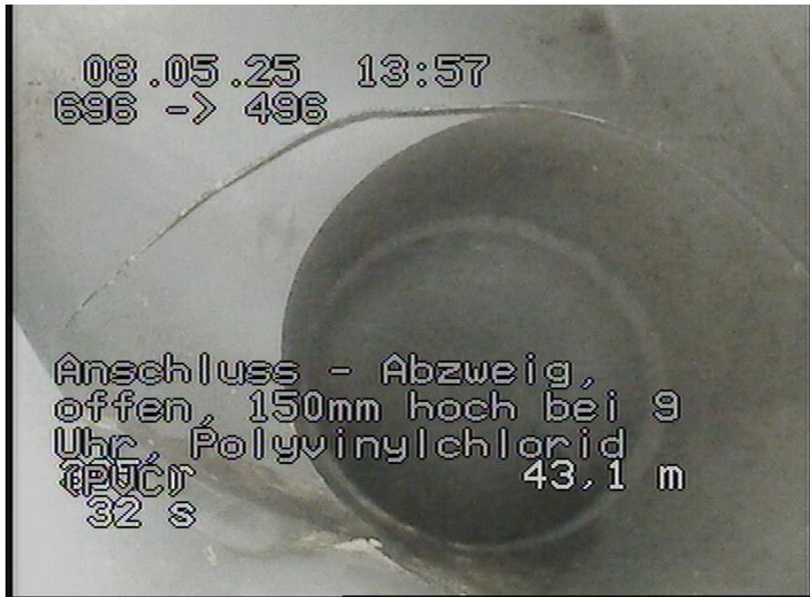
696-496_669.jpg, 00:06:09, 43.10m Anschluss - Abzweig, offen, 150mm hoch bei 9 Uhr, Polyvinylchlorid (PVC)
