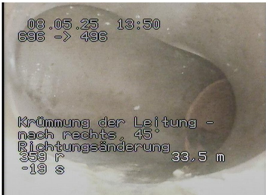
696-496_662.jpg, 00:03:06, 33.50m Krümmung der Leitung - nach rechts, 45° Richtungsänderung
