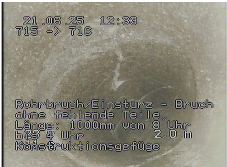
715-716_764.jpg, 00:00:18, 2.00m Rohrbruch/Einsturz - Bruch ohne fehlende Teile, Länge: 1000mm von 8 Uhr bis 4 Uhr / Konstruktionsgefüge zerstört
